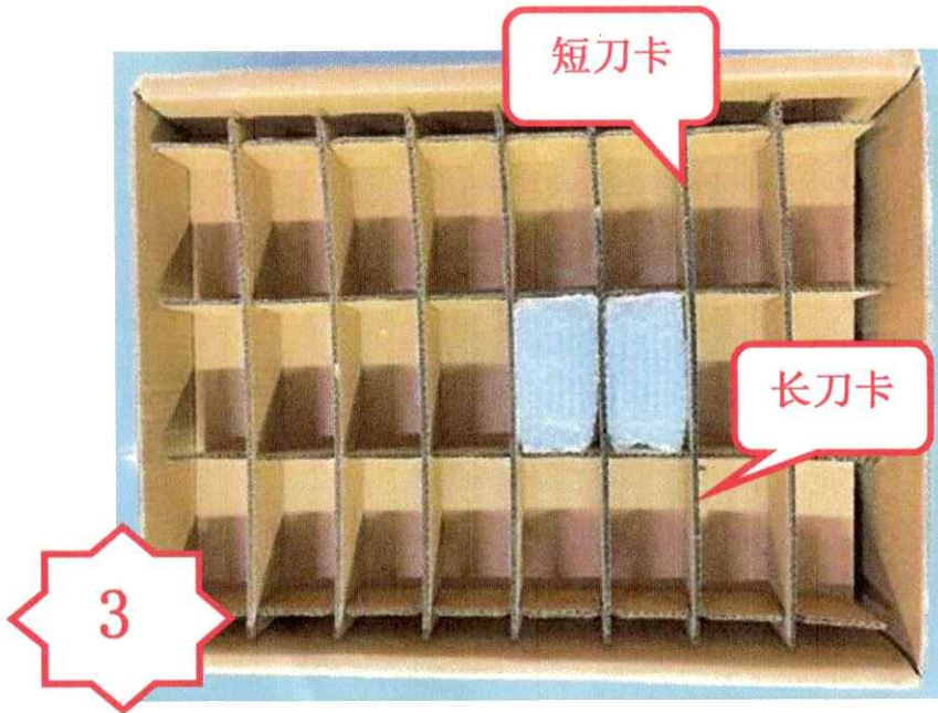
图三，每 1 个气泡袋装 10 个组件，每格放 2 袋 20 个，每层 24 格 480 个，每箱三层的方式包，共 1440 个，同时在底层，顶层各放 1 块隔板，中层 2 块。
